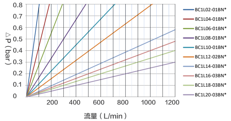
10 \mu\text{m} 流量差压曲线
